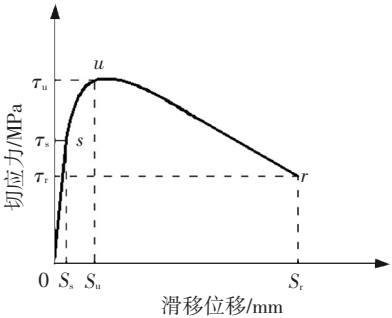
图 8 切应力-滑移位移特征曲线
