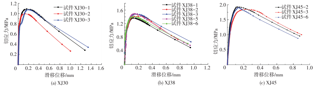
图 7 切应力-滑移位移曲线
