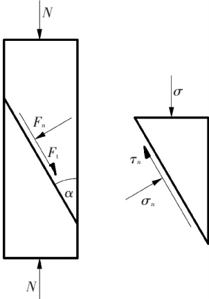
图 5 棱柱体剪切试验应力分析 Fig.5 Stress analysis of SST
