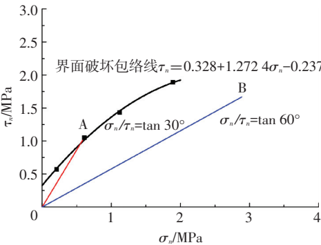
图 6 界面破坏包络线分析
