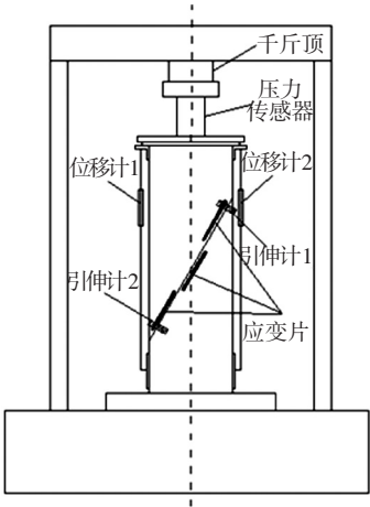
图 3 测点布置
